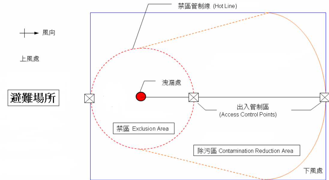
圖 8-6-1、避難場所區域劃分示意圖
